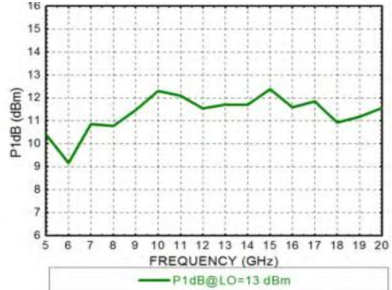
Input P1dB
